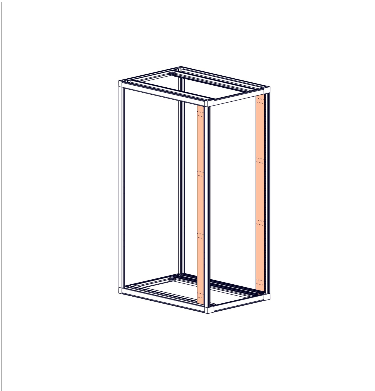
Cabinet airtight sideplates
